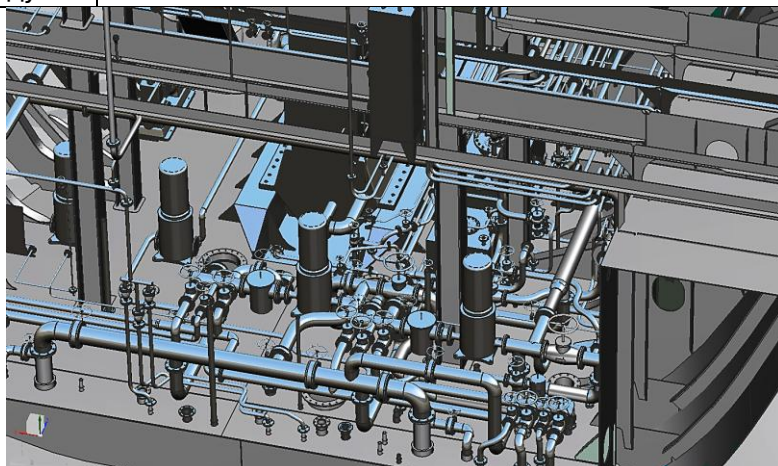
3D модел на машинно отделение с пълно палубно отръбoproводяване
