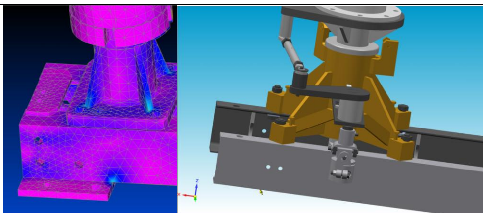
Зони с максимално натоварване и оптимизиране на кинематична схема
