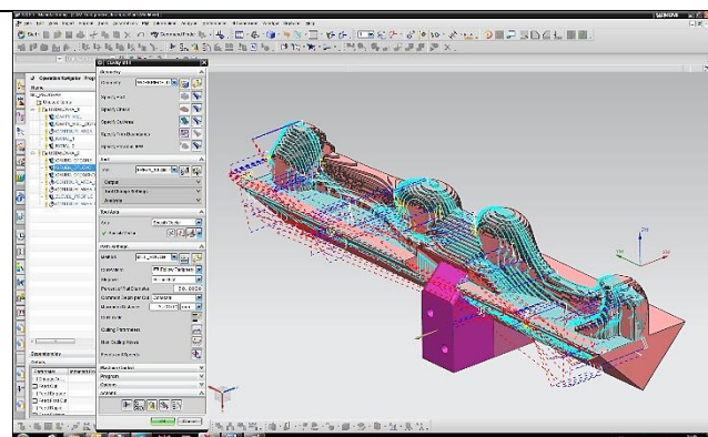
Симулация на постпроцесори с визуализация от G-кода след пост процесора
