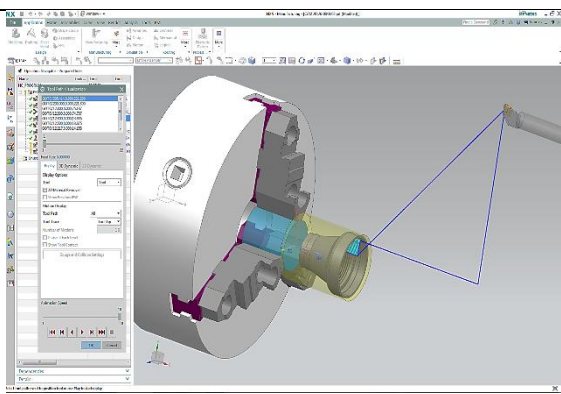
Симулация на постпроцесори с визуализация от G-кода след пост процесора
