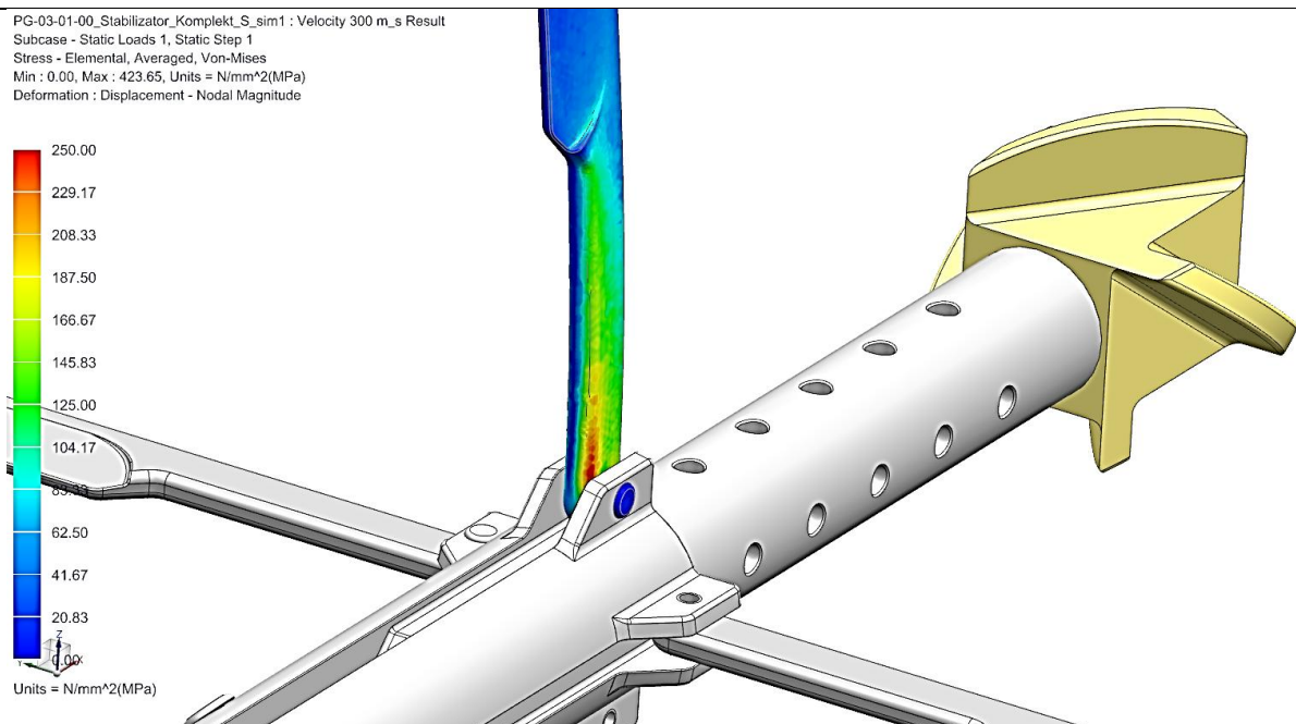
Оценка на напрежение/деформации при движение във флуидна среда
