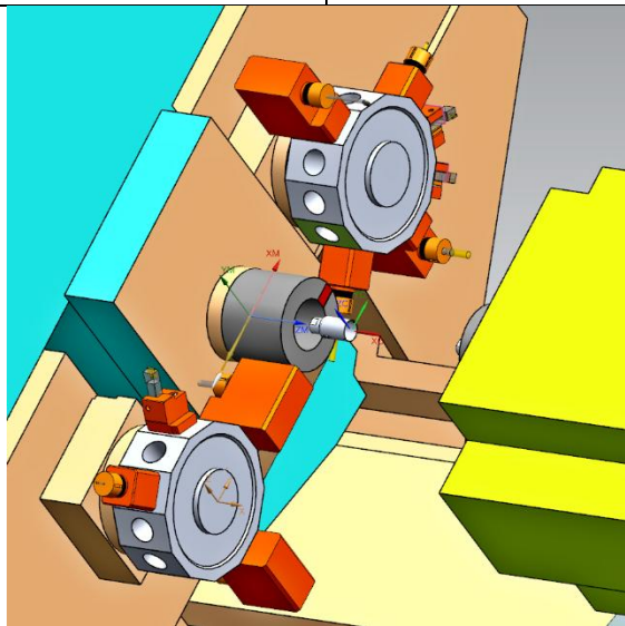
САМ постпроцесор за Самел 90
