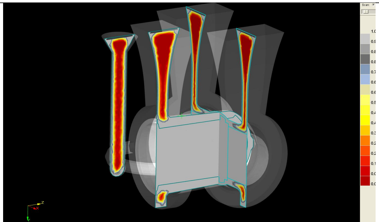
Солидификация - позициониране на мъртви глави
